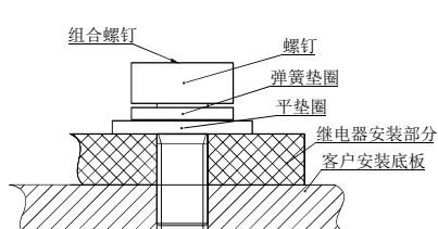
继电器安装
