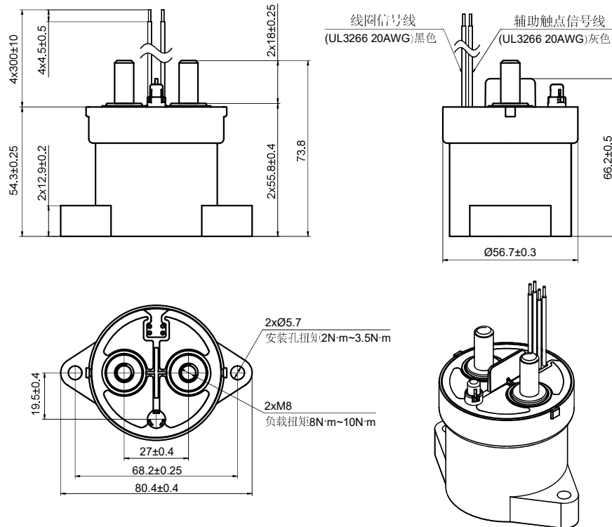
HFZ21-300 外螺纹
