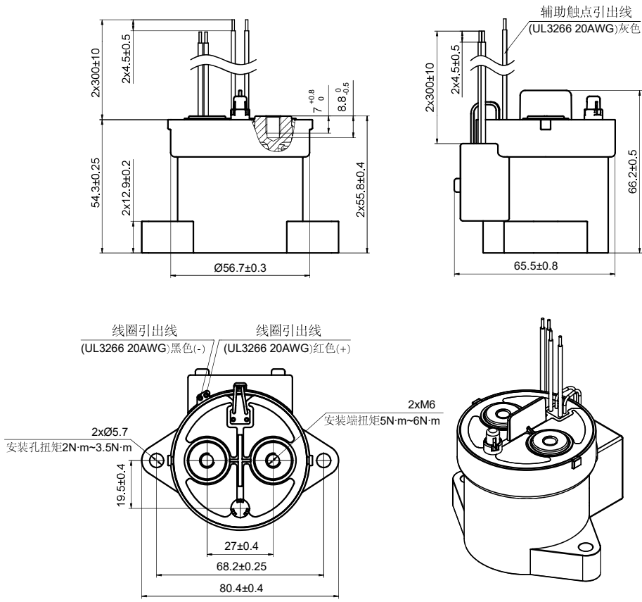
HFZ21-250-B内螺纹
