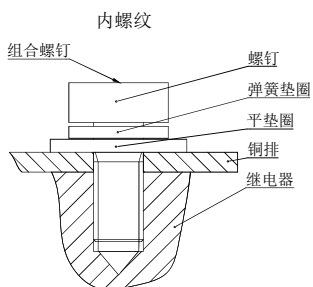
负载端安装
